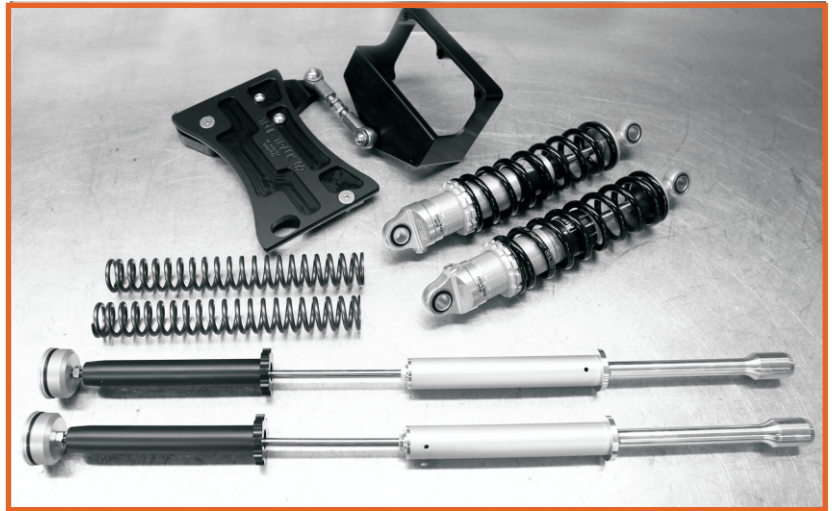
Fahrwerksskit von G&R
